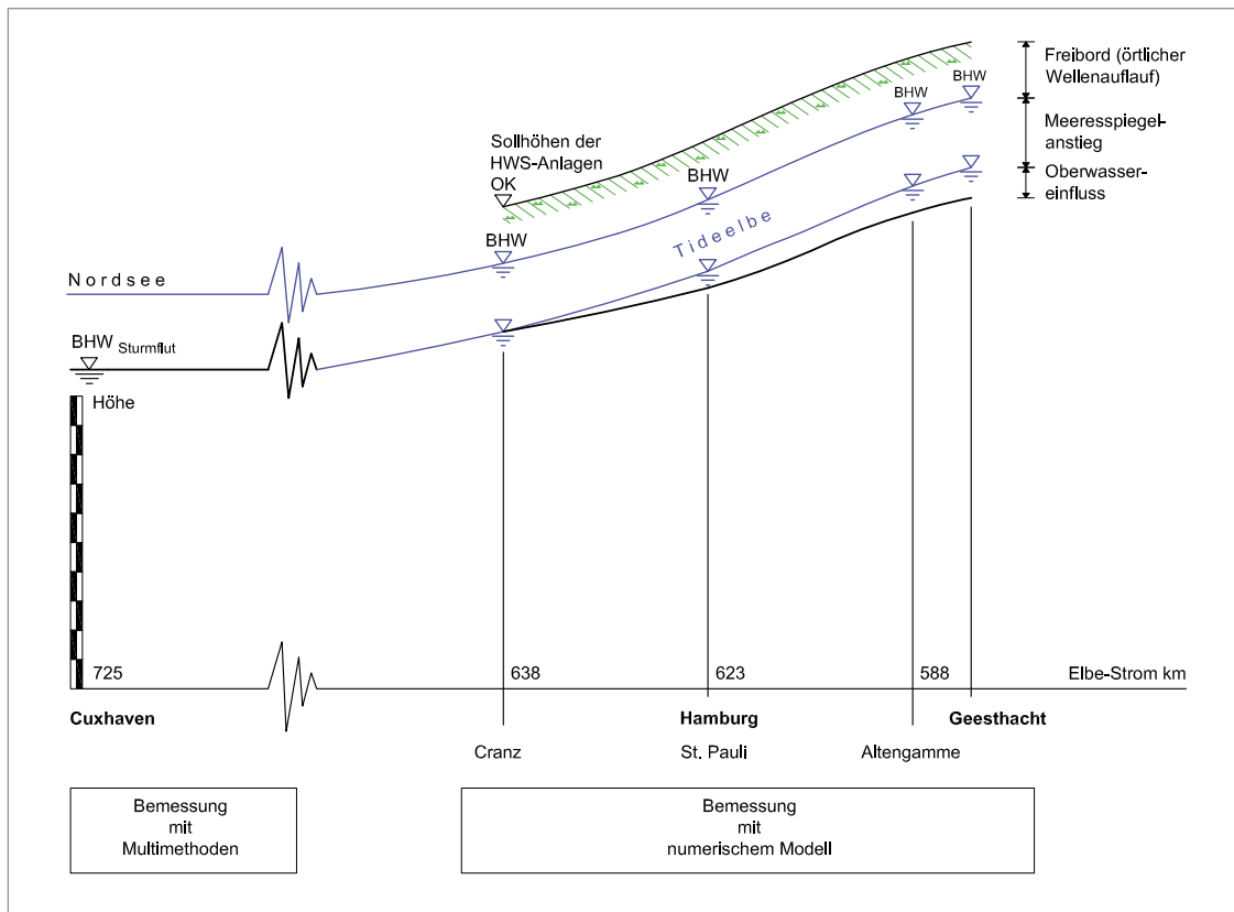
Abb. 2-2: Bemessung in der Tideelbe
