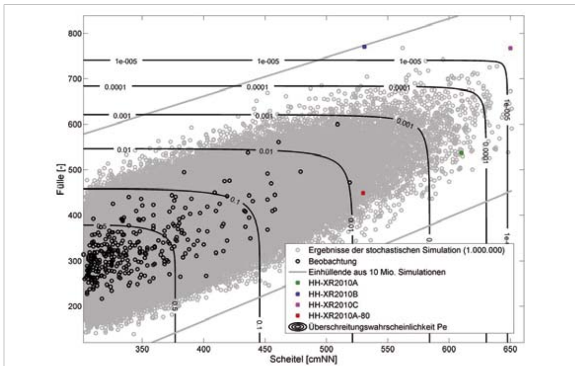
Abb. 2.2-3: Zweidimensionale Extremwertstatistik (Wahl et al., 2012)
