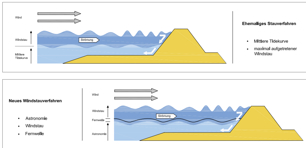
Abb. 2.1-4: Vergleich der Staukurvenanalyse und der Windstaukurvenanalyse
