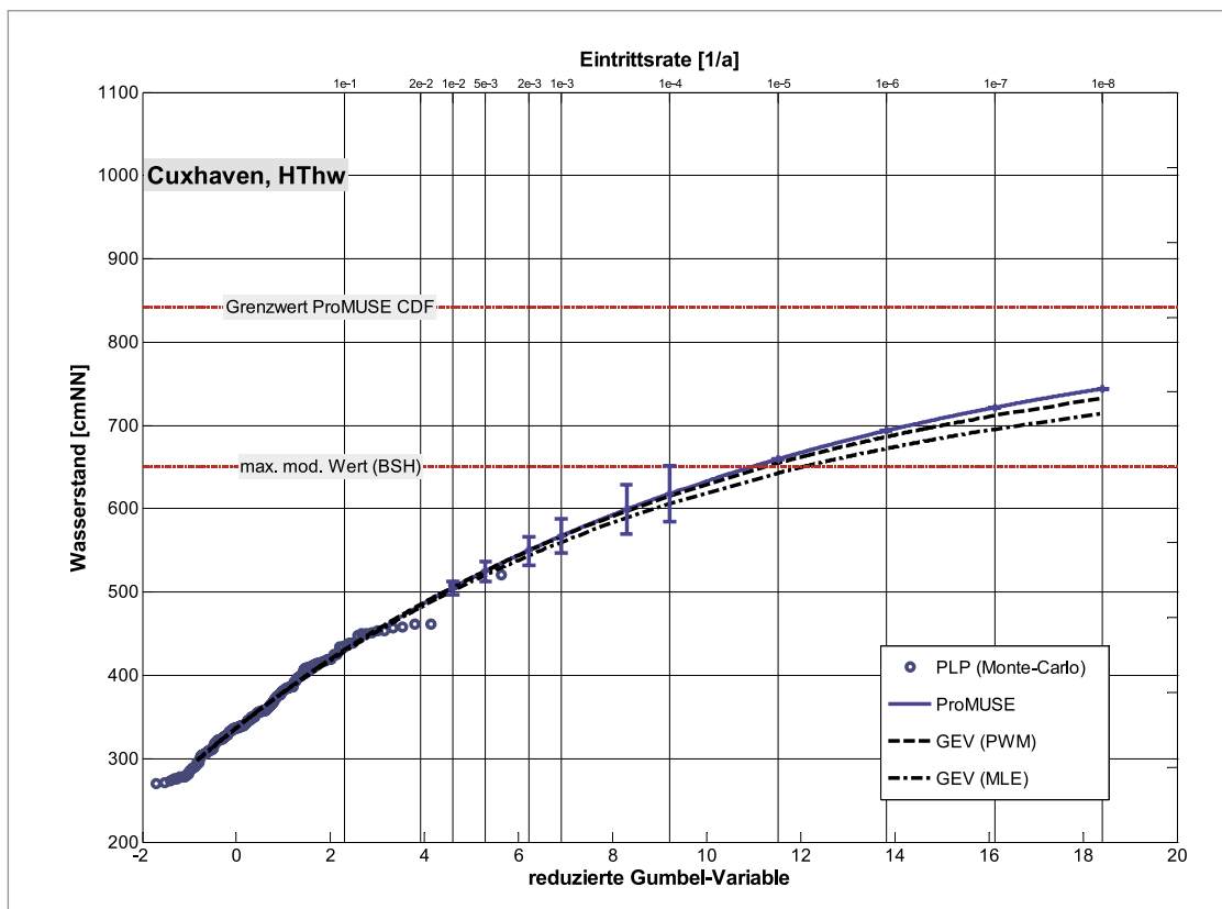
Abb. 2.2-1: Prinzipskizze der integrierten Extremwertverteilung mit beobachteten und modellierten Daten am Beispiel der Cuxhaven (Jensen et al., 2005)
