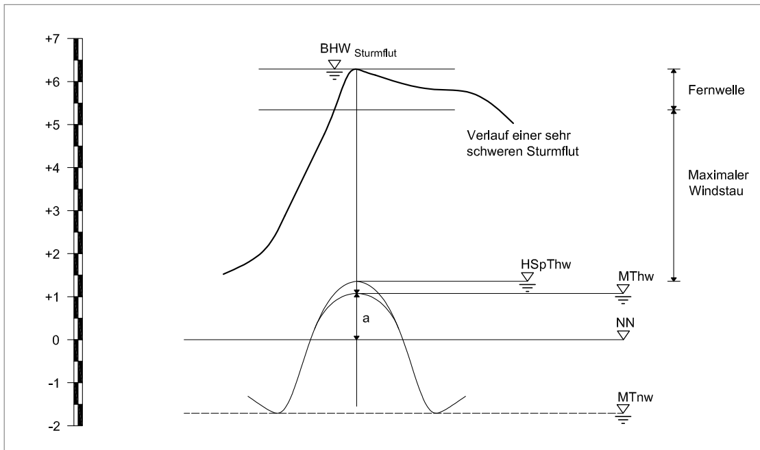
Abb. 2.1-5: Die Bemessungsturmflut unter Berücksichtigung nicht-linearer Effekte (Windstaukurvenanalyse)
