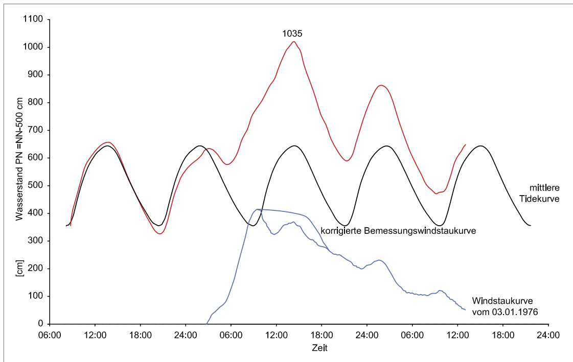
Abb. 2.1-3: Staukurvenanalyse am Pegel Cuxhaven
