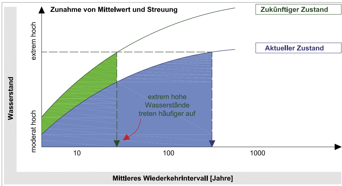
Abb. 2.2-2: Instationäre Extremwertstatistik (Mudersbach , 2009)
