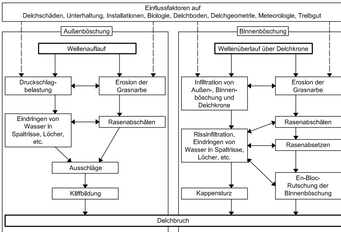
Abb. 2.2-4: Ursachen eines Deichbruches durch Versagensmechanismen auf der Außen- und Binnenböschung von Deichen (Oumeraci und Schüttrumpf, 1997)
