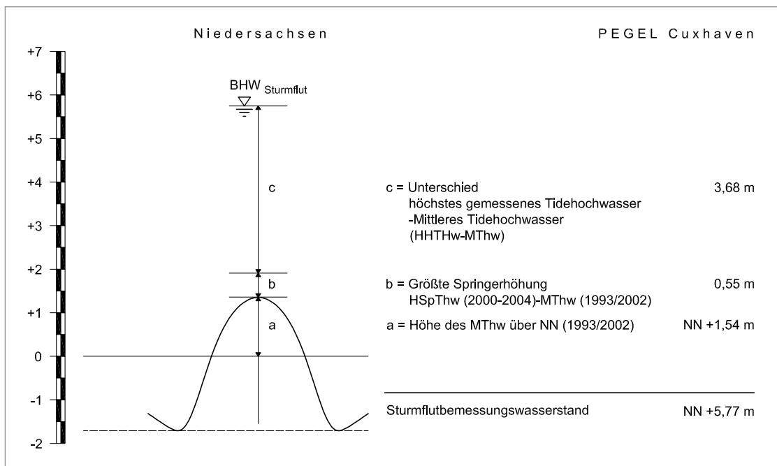
Abb. 2.1-2: Das in Niedersachsen und in der Hansestadt Bremen verwendete Einzelwertverfahren
