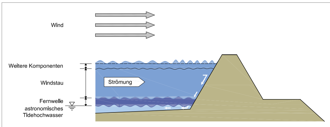
Abb. 2.1-1: Komponenten einer Sturmflut
